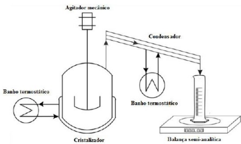
Aparato experimental de cristalização evaporativa por batelada
