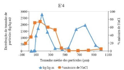
Gráfico obtido por argentometria
