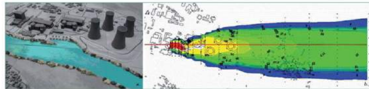
Figure 1: Expérimentation en soufflerie - a : modèle physique de la centrale ; b : champ d'activité mesuré au sol.
